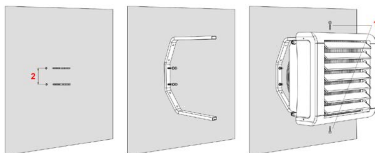
Рис. 4. Монтаж консоли
